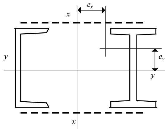
Рис. 6. Сквозное сечение стержня из двух сплошнотенчатых ветвей
